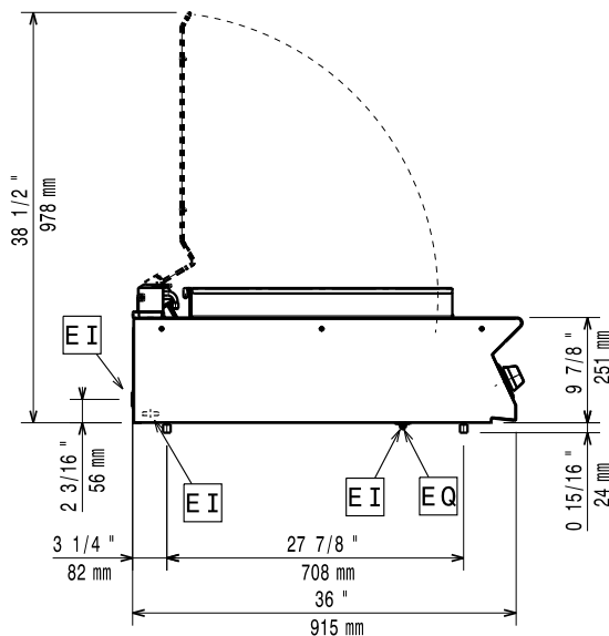
Zij aanzicht
